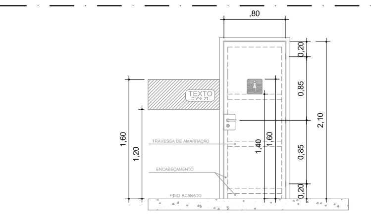
DET. GENÉRICO - SINALIZAÇÃO TÁTIL E VISUAL ESC.: 1:50
